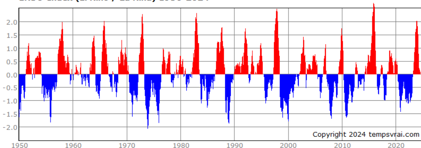
ENSO-Index (El Niño / La Niña) 1950-2024
