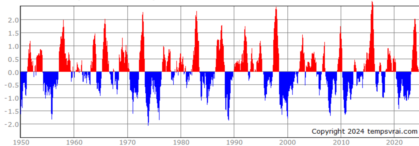
ENSO-Index (El Niño / La Niña) 1950-2024
